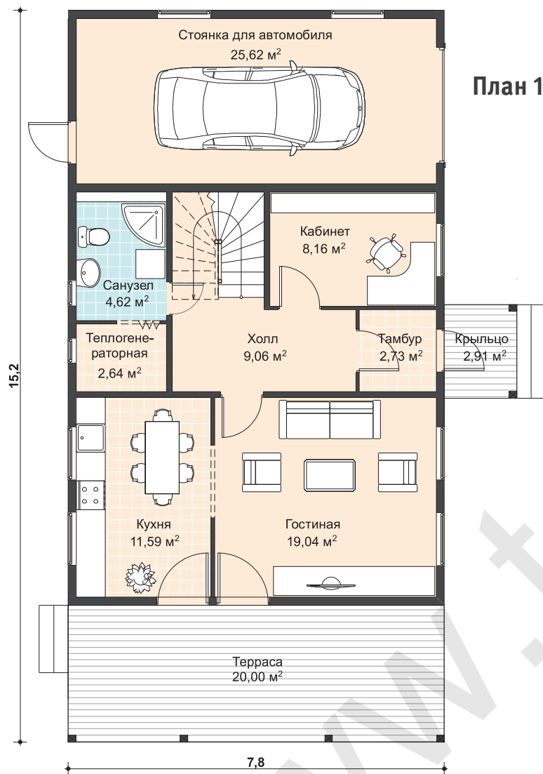
План 2 этажа
