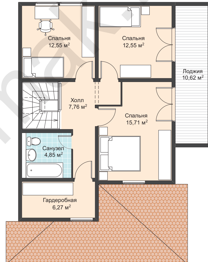
План 2 этажа
