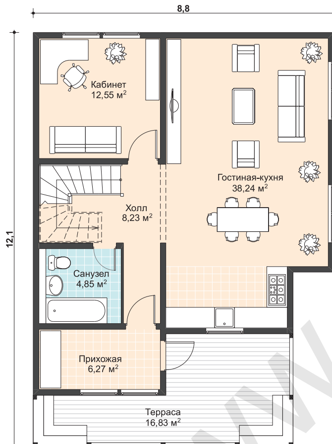
План 1 этажа
